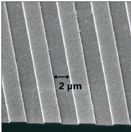
Réseau de phases d'une hauteur d'env. 0,25\text{ }\mu\text{m}
