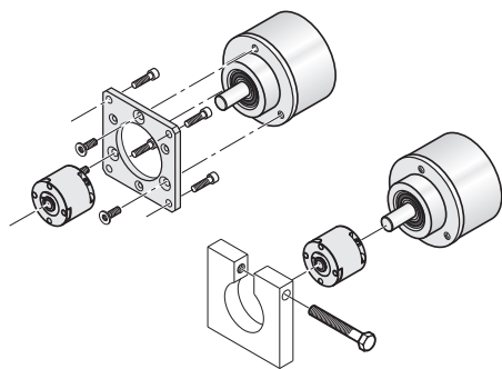
Bride de serrage
