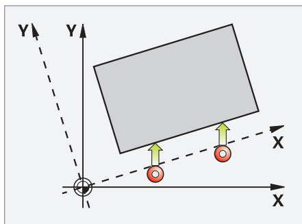
Compensation de l'erreur d'alignement par une rotation de base du système de coordonnées ou par une rotation du plateau circulaire
