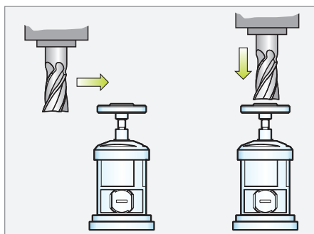
Étalonnage d'outils par ex. de la longueur et du rayon de l'outil ou de l'usure de l'outil
