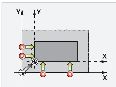
Définition du point d'origine par ex. au niveau d'un coin ou au centre d'un cercle de trous
